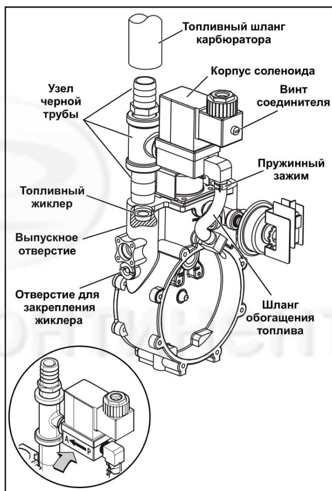
Рис. 2-3. Сборка регулятора подачи
